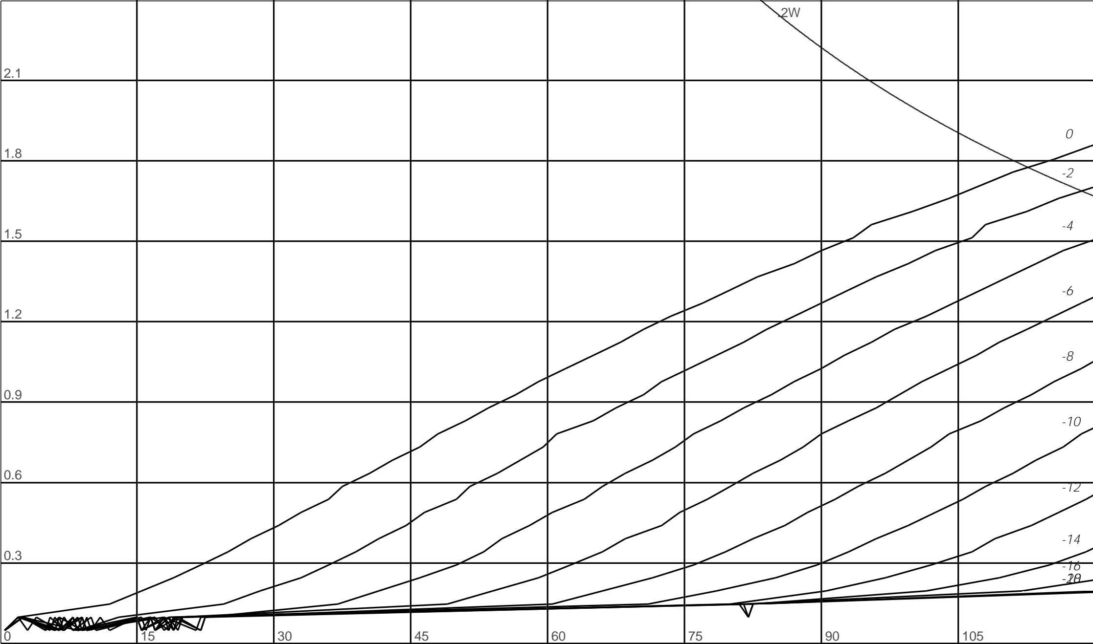
VT1 Ua : 0 à 120V, Filament: 2V
