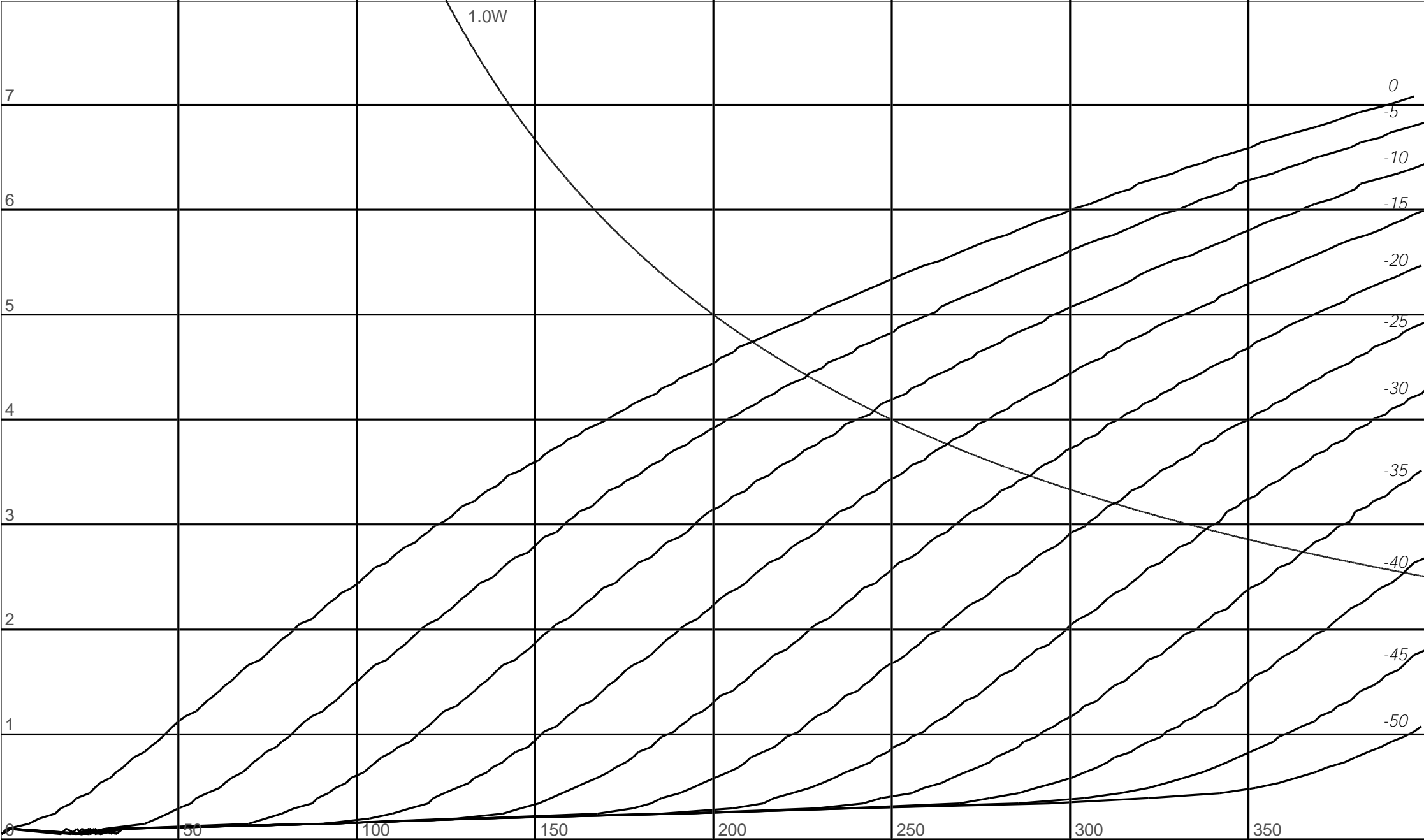
VT1 U_a :0 à 400 V, Filament: 2,2 V
