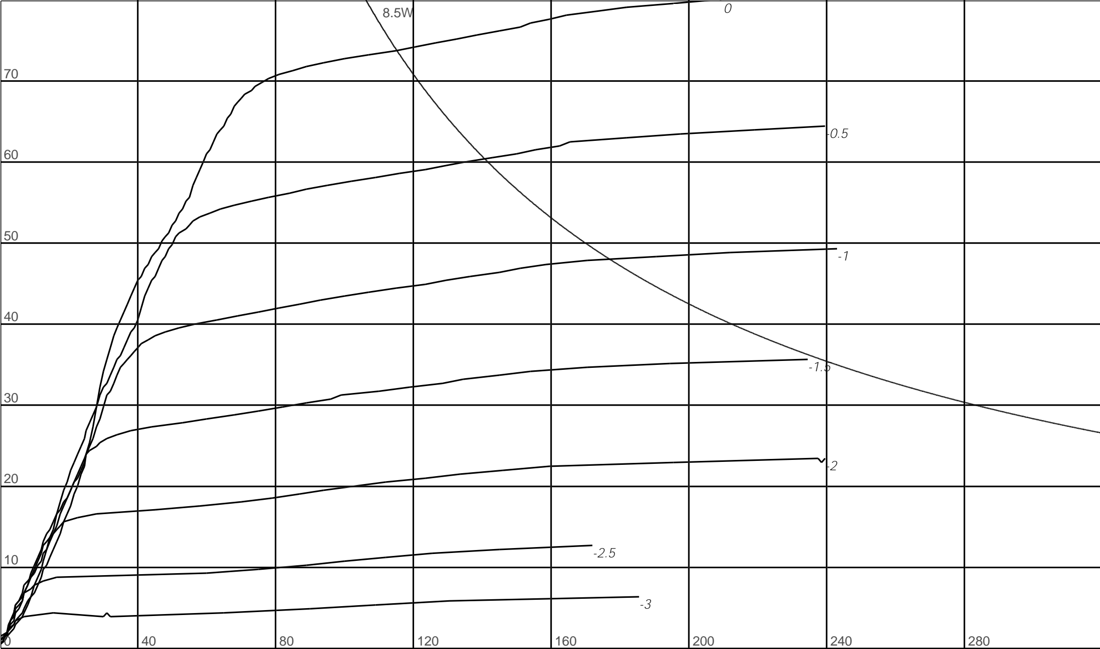
WE418A-1 Penthode (pour vérif)
