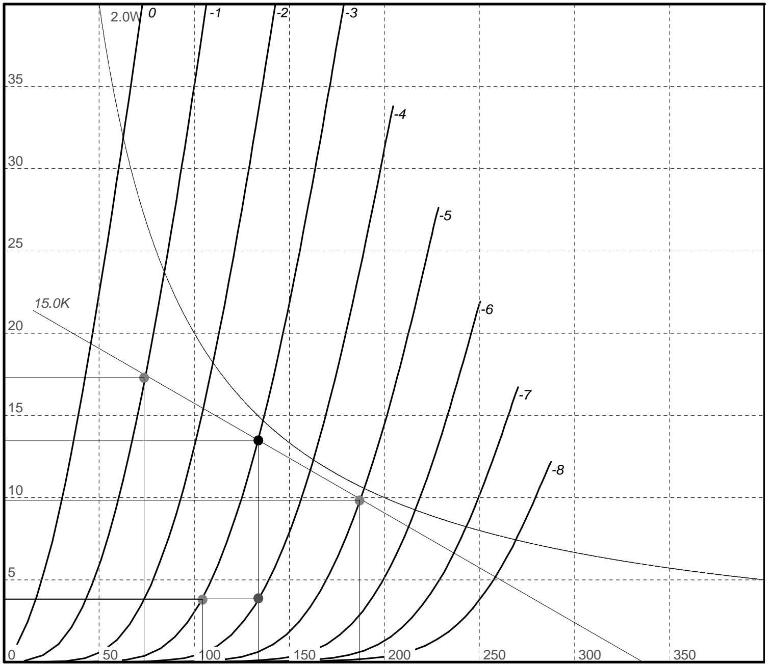
ECC88. 134V, 14mA.
