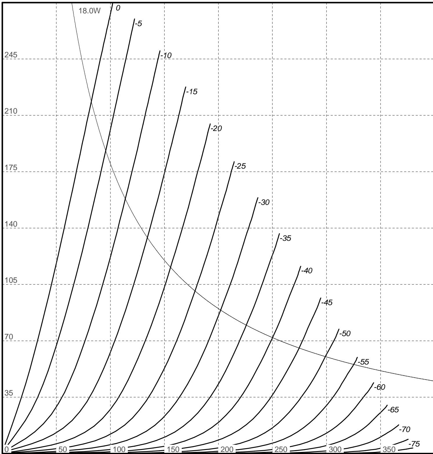
EL36-115. Mode triode.
